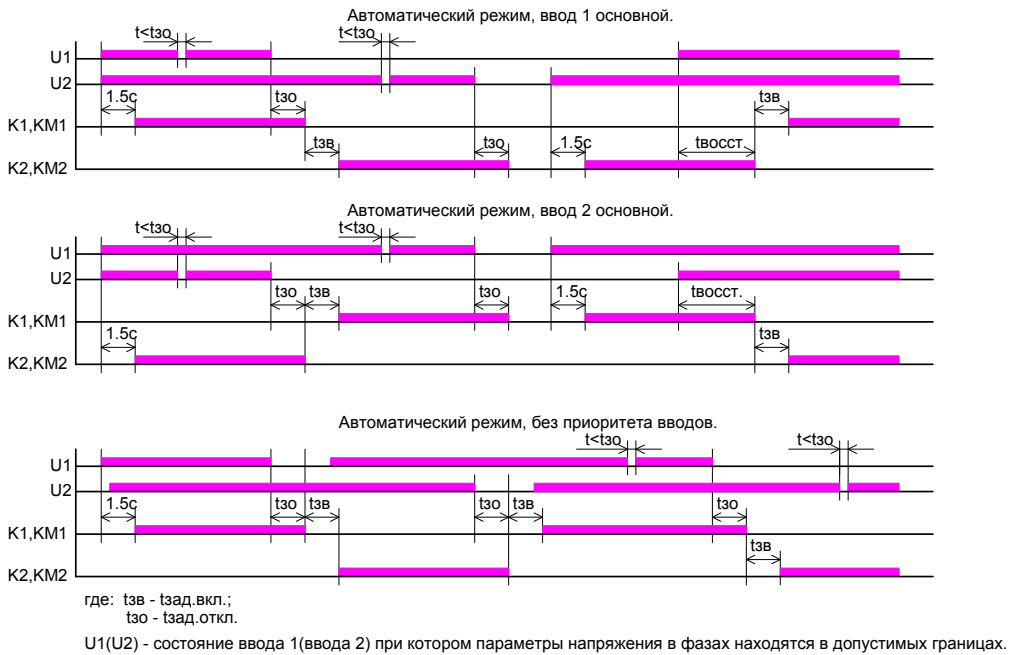
Рис.3 Схема и временные диаграммы работы АВР на магнитных пускателях с двумя вводами, одной группой нагрузок, с электрической блокировкой магнитных пускателей и управлением от БУАВР1.х.х
