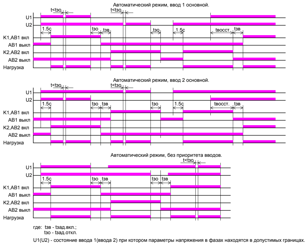
Рис.4 Схема и временные диаграммы работы АВР на автоматических выключателях с мотор-приводом, двумя вводами, одной группой нагрузок, электрической блокировкой автоматических выключателей и управлением от БУАВР1.х.х. Схемы получения оперативного питания представлены в разделе 5 настоящего РЭ.
