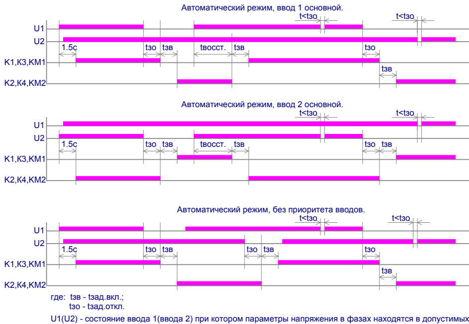
Рис.3 Схема и временные диаграммы работы АВР на магнитных пускателях с двумя вводами, одной группой нагрузок, с электрической блокировкой магнитных пускателей и управлением от БУАВР.К.х.х
